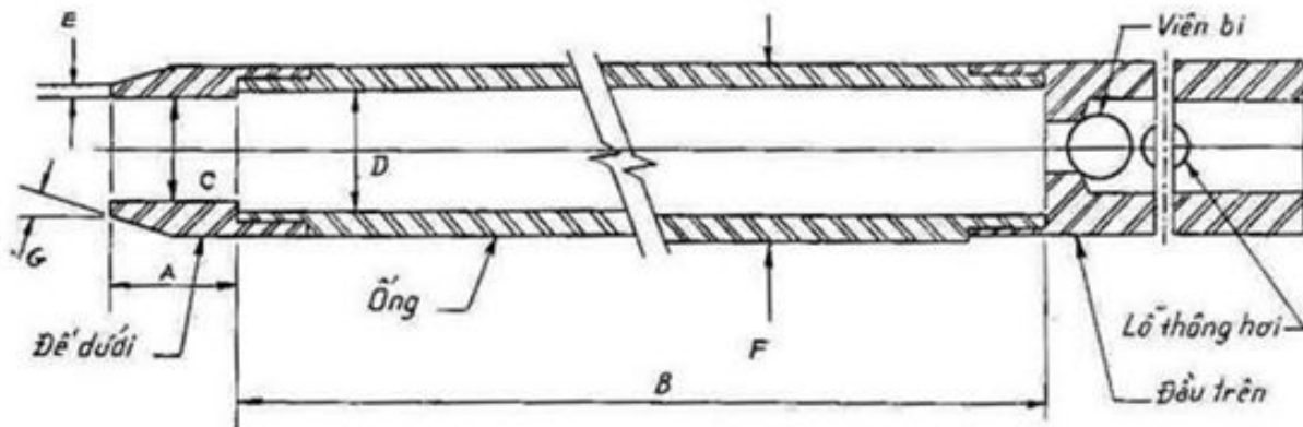
Hình 3: Mũi xuyên SPT
