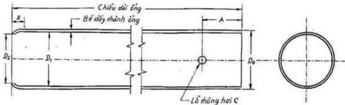
Hình 2: Ống lấy mẫu thành mỏng
